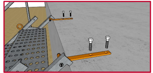
Befestigung an der Deckenkante mit bau-seitigen Schwerlastankern
