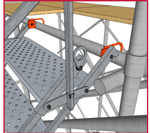
Befestigung am Gerüst mit angebrachten Haken
